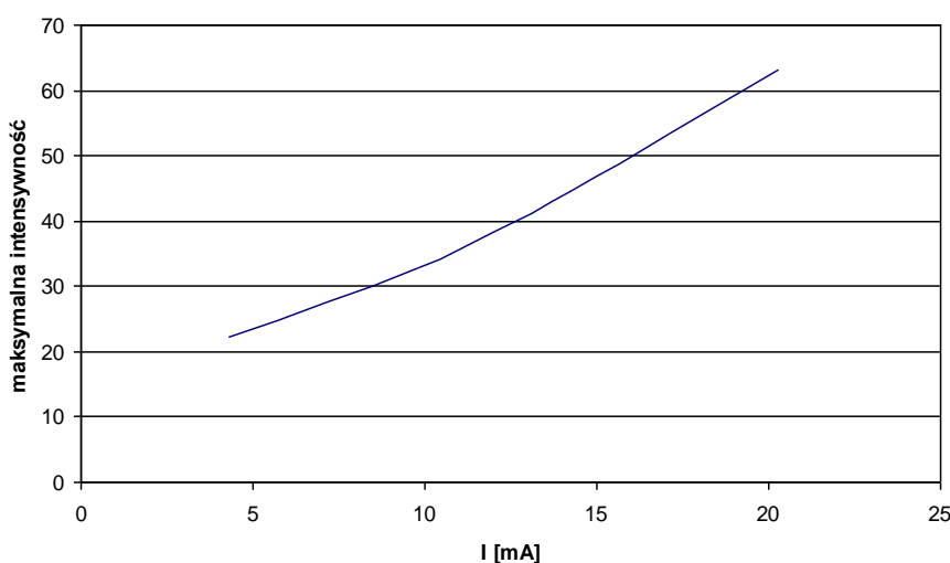
Rys. 3.3 Przykładowa charakterystyka intensywności w funkcji prądu – dioda żółta.
