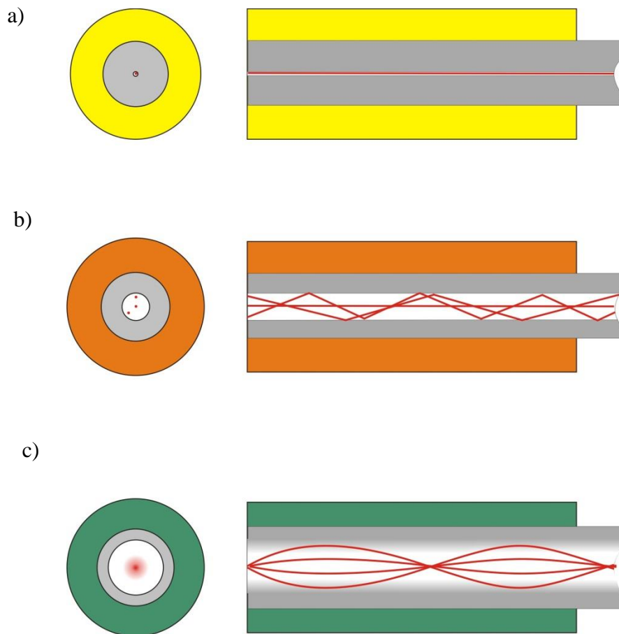
Rys. 1.4. Teoretyczna droga poruszania się impulsu świetlnego w światłowodzie (a) jednomodowym, (b) i (c) wielomodowym.
