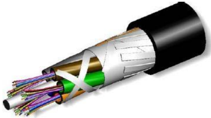
Rys. 1.7 Kabel wielotubowy
